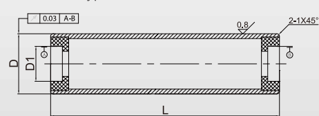
无轴型 Without shaft type
