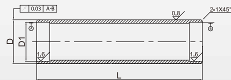
无轴型 Without shaft type
