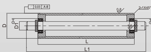
带轴型 Shaft type
