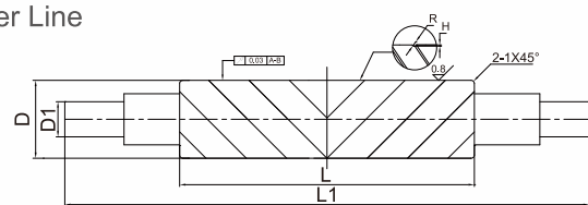
中心开线 Center Line
