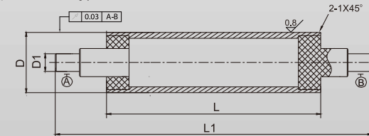
带轴型 Shaft type
