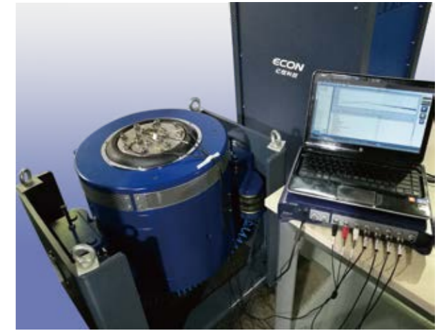
· 振动台检定装置 Vibration table verification device
